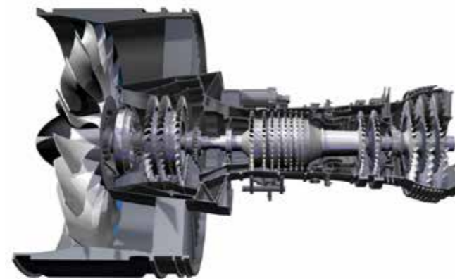
PW1100G-JMの開発のベースとなるPW1000G (P&W)
